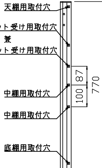
支柱取付穴詳細図
