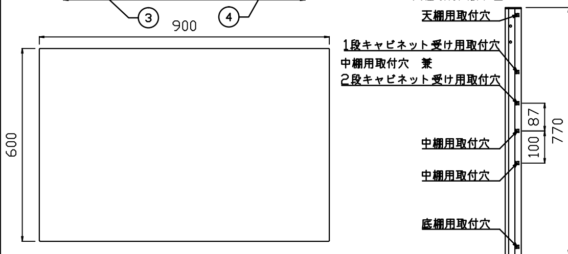
支柱取付穴詳細図
