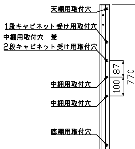
支柱取付穴詳細図
