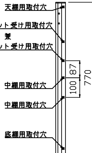
支柱取付穴詳細図
