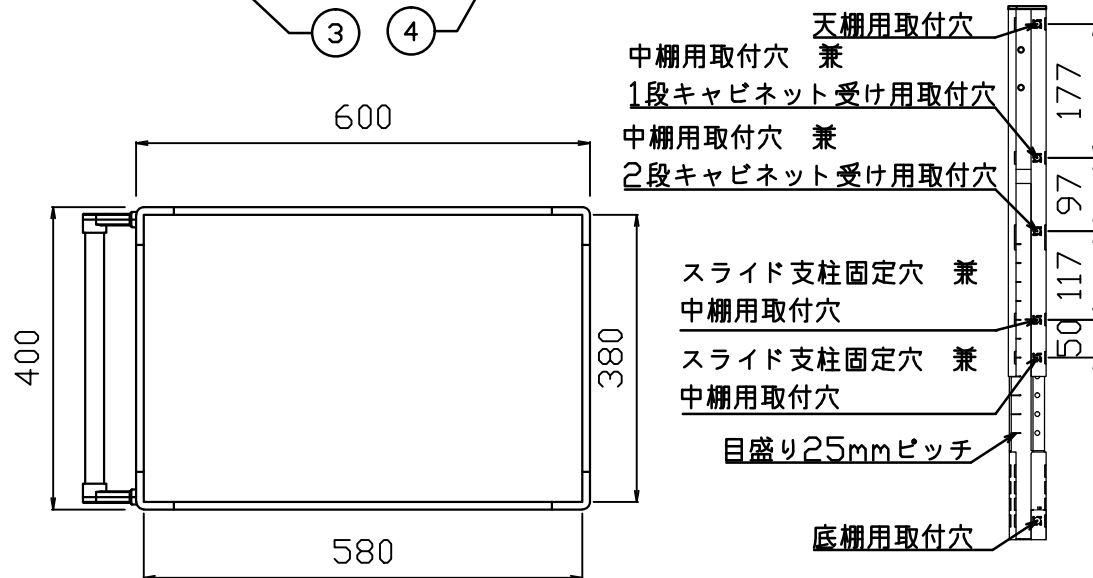
支柱取付穴詳細図
