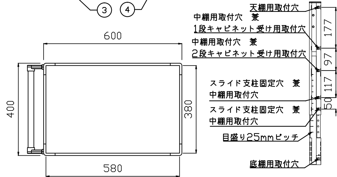
支柱取付穴詳細図
