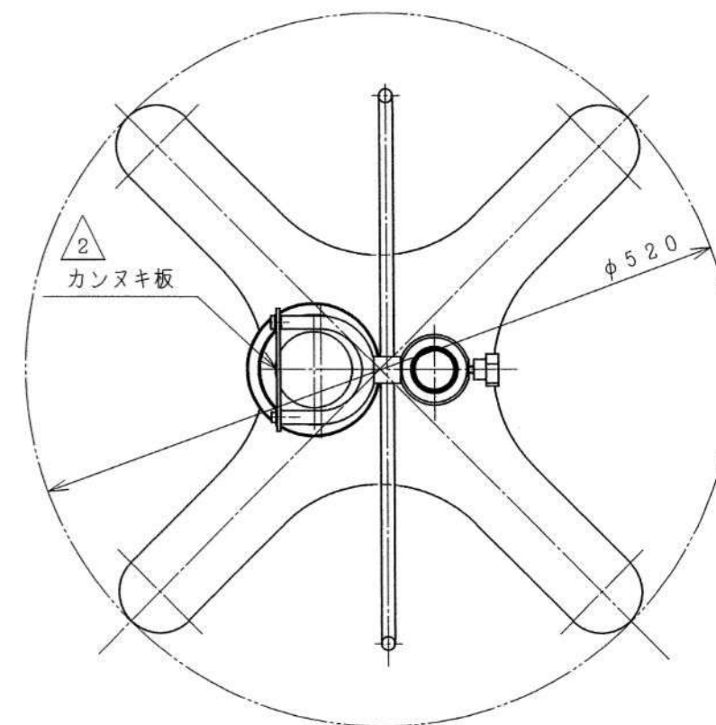
A 矢視
