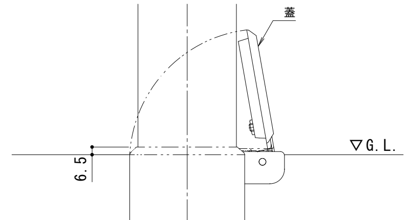
埋設管蓋部詳細図 S = 1 : 3
