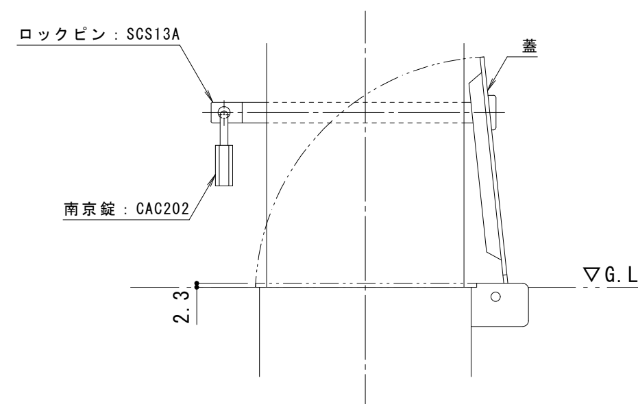
南京錠部詳細図 S = 1 : 3
