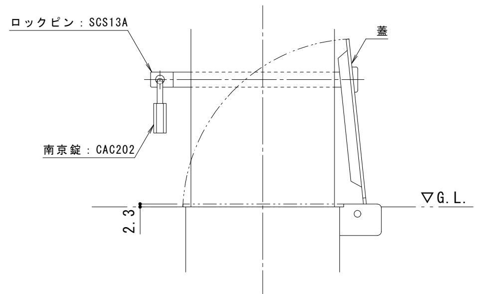
南京錠部詳細図 S = 1 : 3
