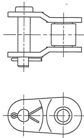
オフセットリンク
