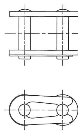
継手リンク(クリップ形)
