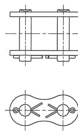
継手リンク(割ピン形)
