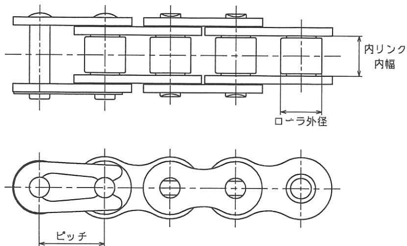
リベット形
