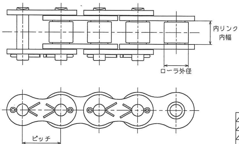
コッター形
