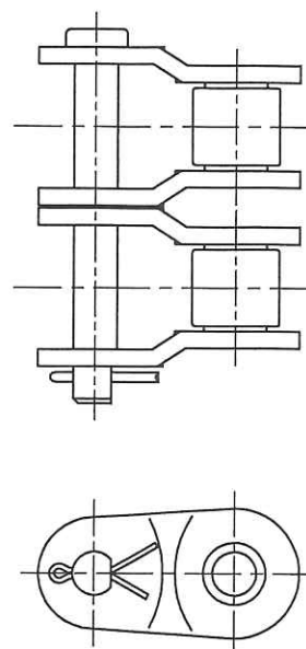
オフセットリンク
