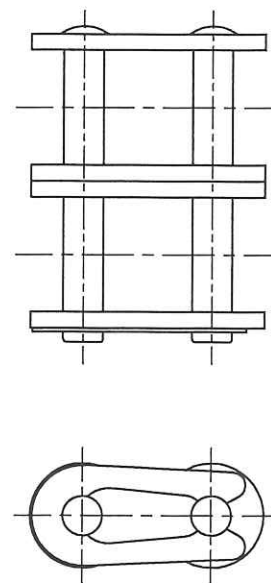
継手リンク (クリップ形)
