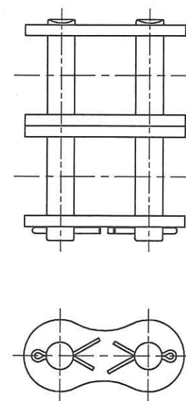
継手リンク (割ピン形)
