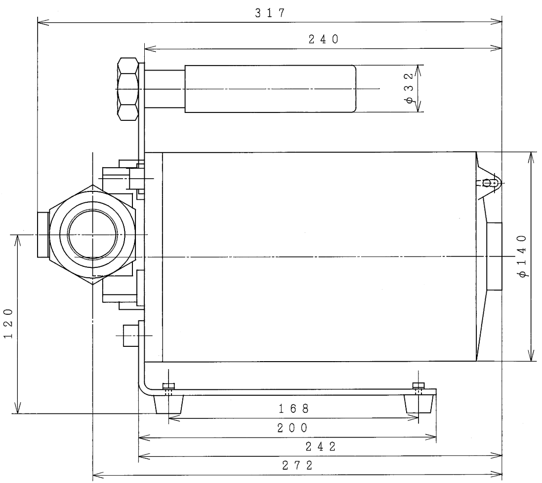
A矢視図 (スケール1:2.5)
