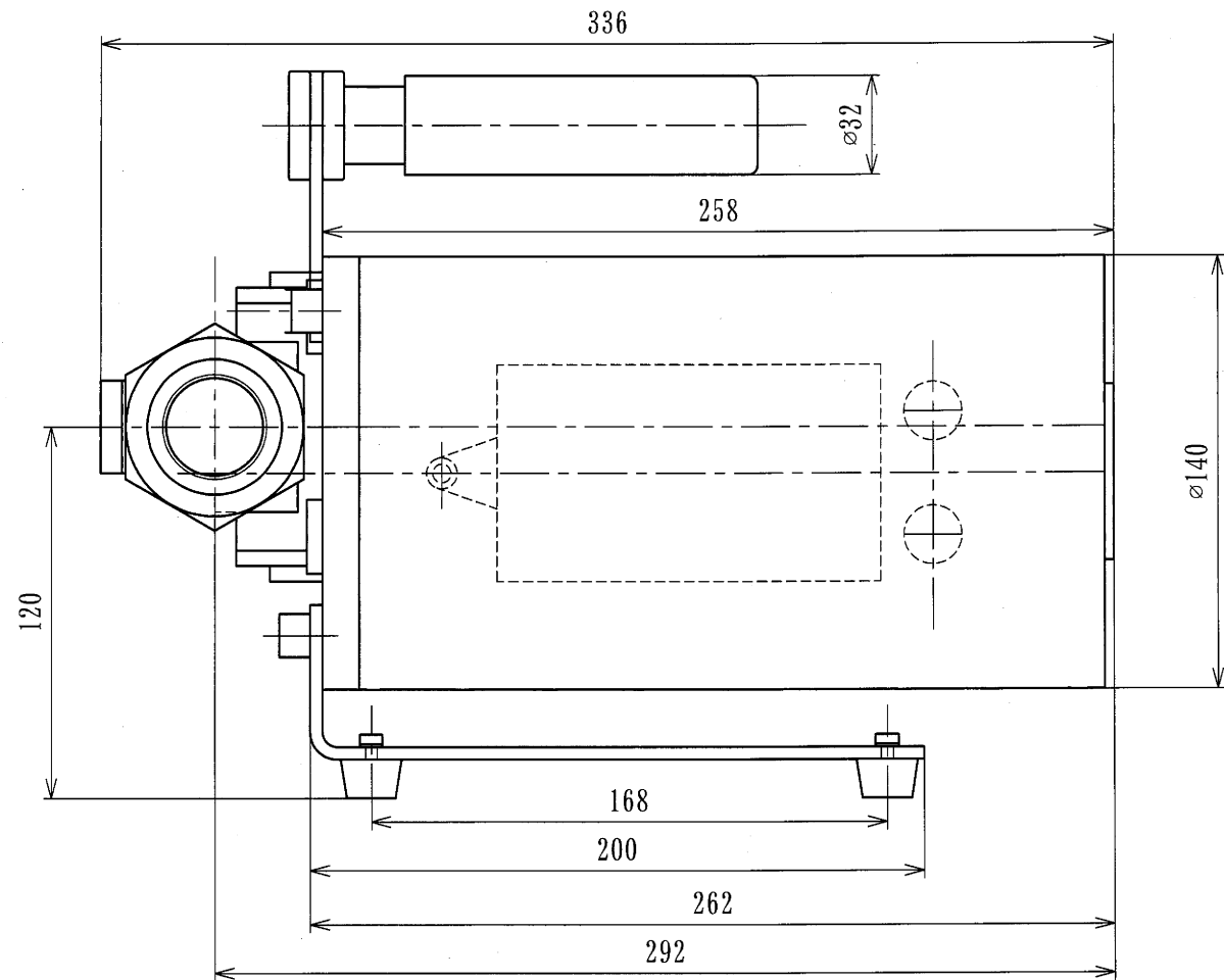
A矢視図 <S=1:2.5>
