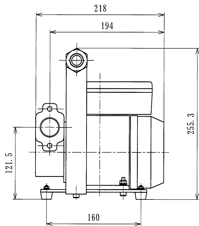
A矢視図
