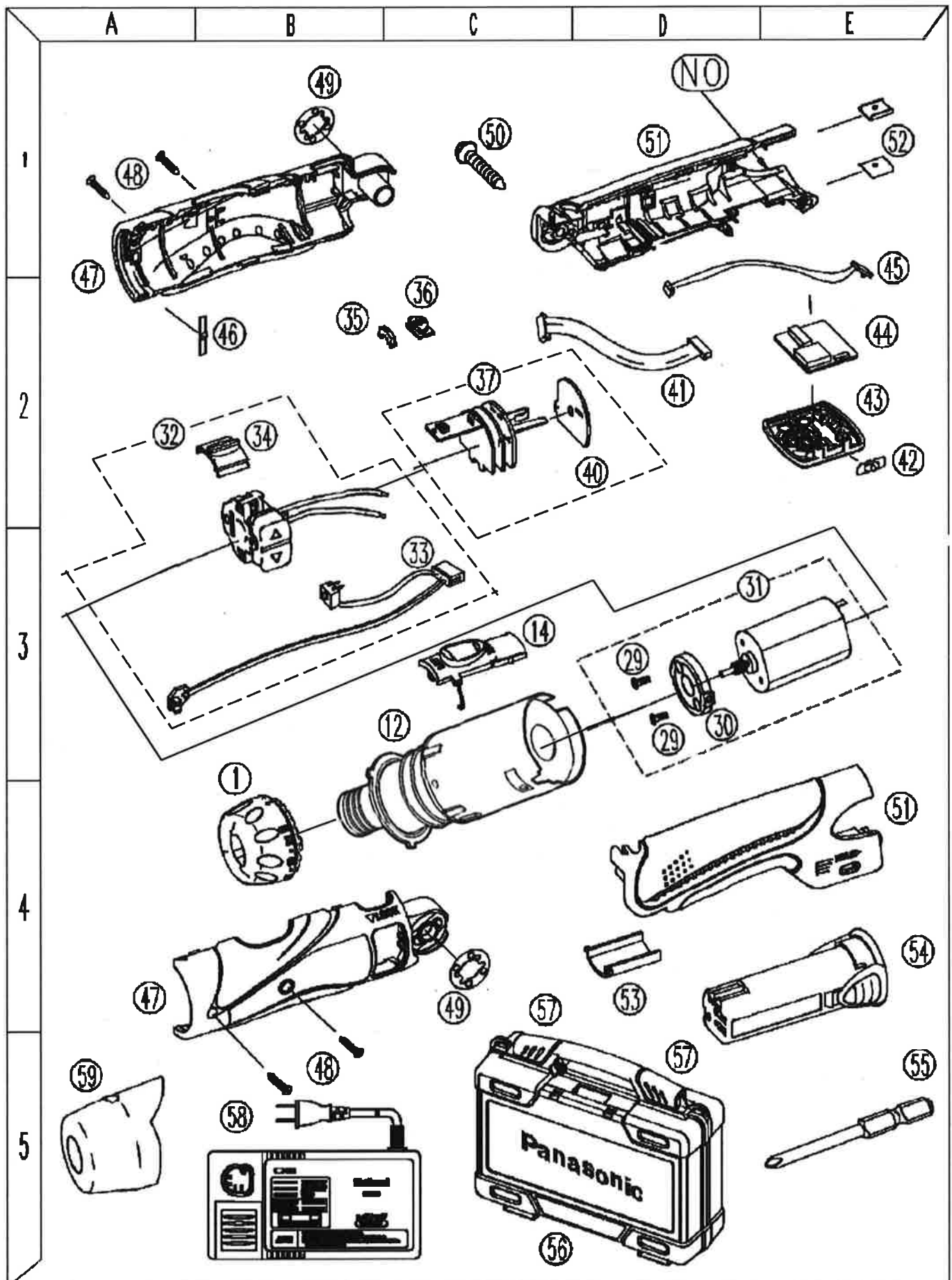
EZ7411-部品展開図
