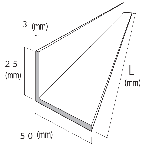
FA143 不等辺アングル
