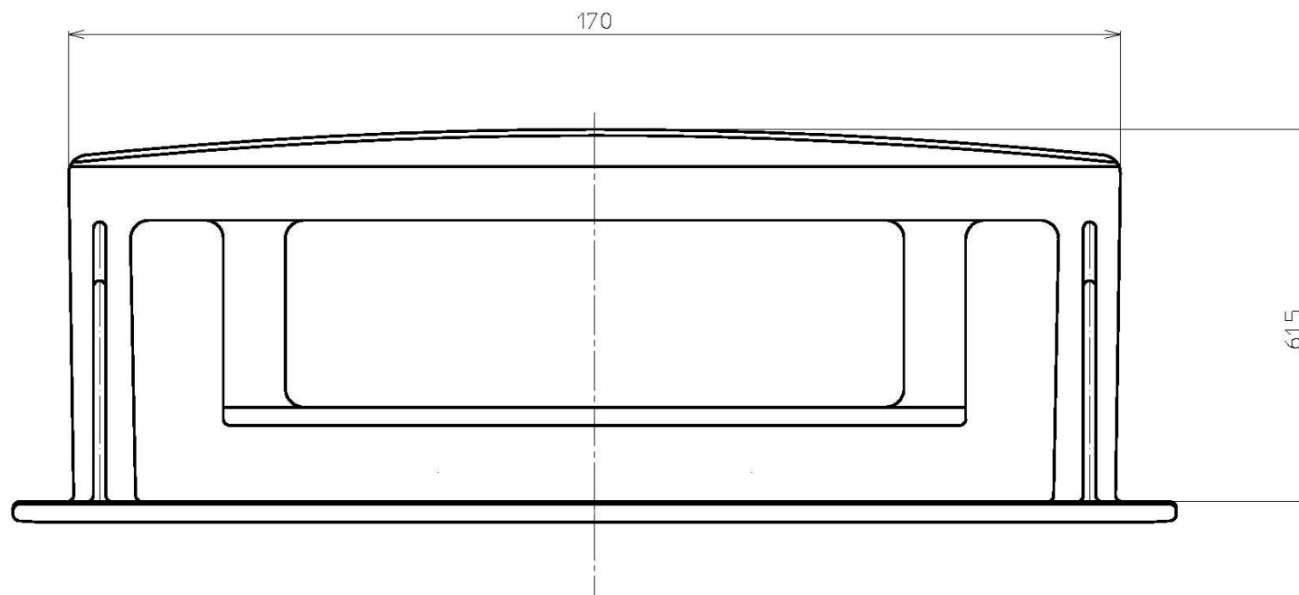
正面図
