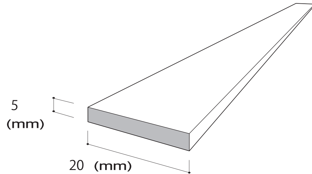
FD109 フラットバー
