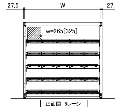
正面図 5レーン
