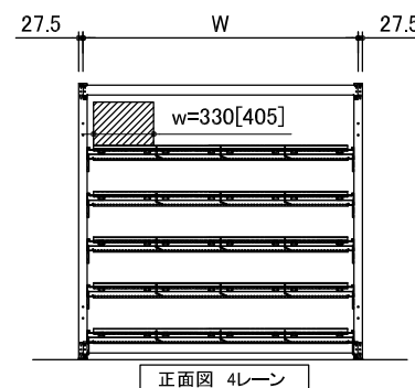
正面図 4レーン
