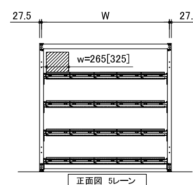
正面図 5レーン
