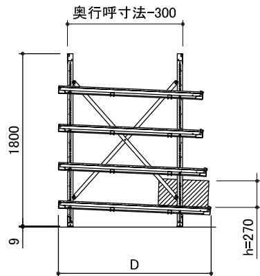
A-A'断面図 奥行1500/1800タイプ
