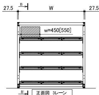
正面図 3レーン
