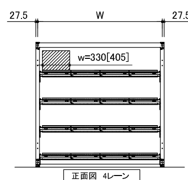
正面図 4レーン
