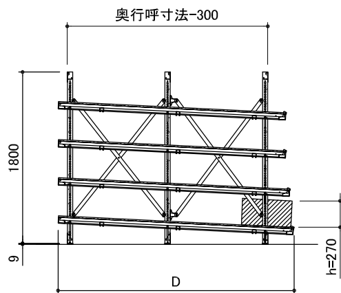
B-B'断面図 奥行2100/2400タイプ
