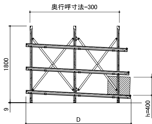
B-B'断面図 奥行2100/2400タイプ
