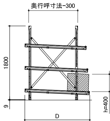
A-A'断面図 奥行1500/1800タイプ
