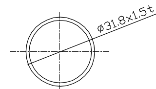
支柱形状
