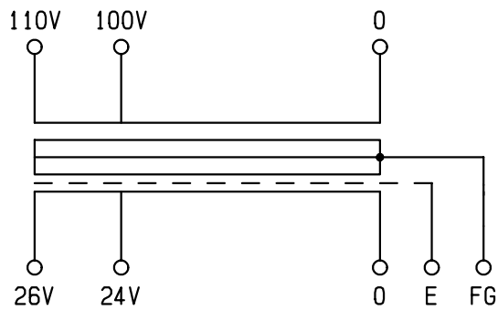
結線図
