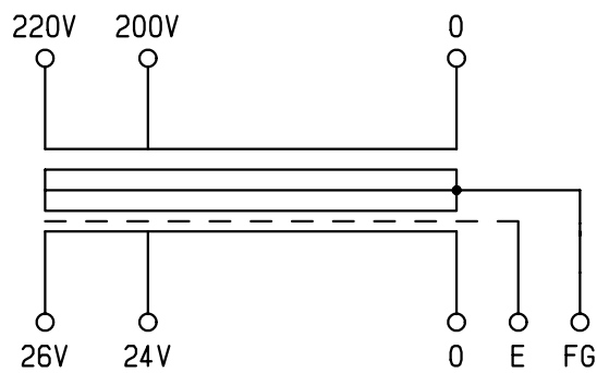
結線図
