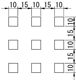
パンチング孔詳細図
