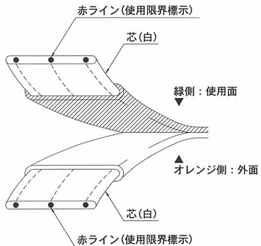
構造図
