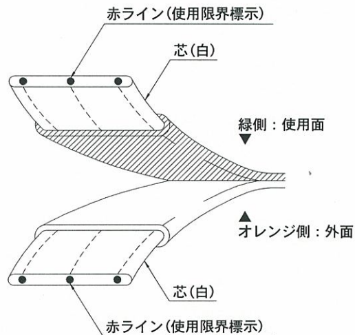
構造図
