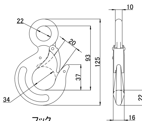
フック
