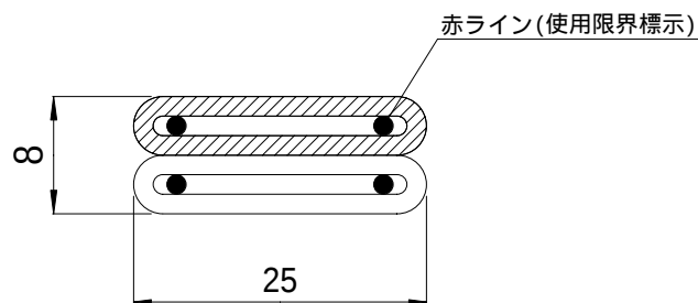
本体部断面
