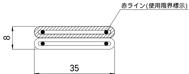
本体部断面
