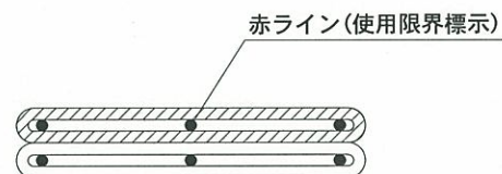
本体部断面
