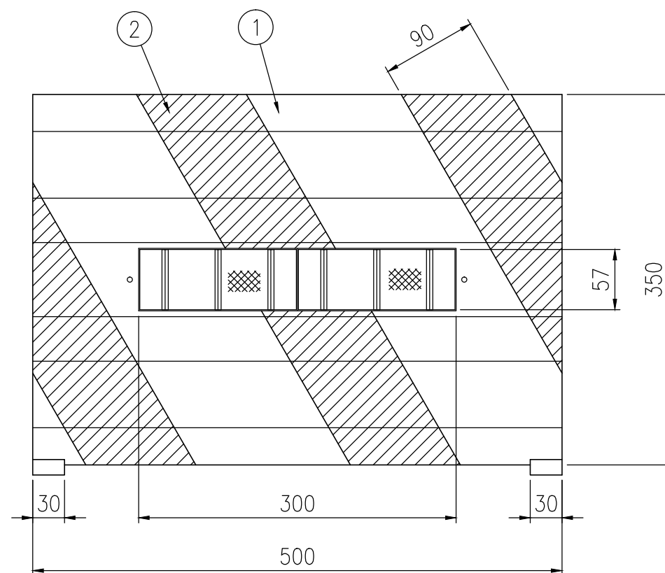
姿図 S=1/5
