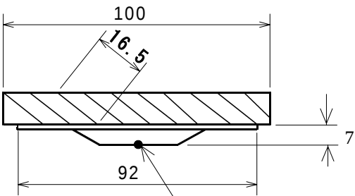
ガラス基盤 穴径 = 16mm 厚さ = 2.5mm
