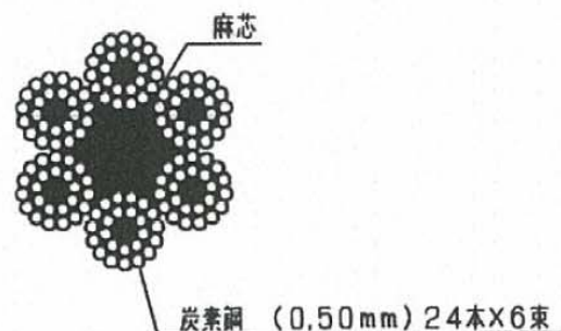
ワイヤーロープ断面図
