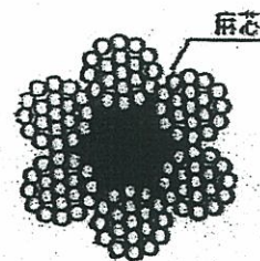
ワイヤーロープ断面図
