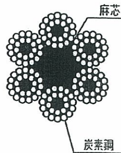
ワイヤーロープ断面図
