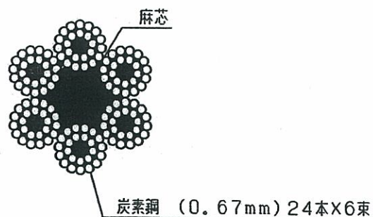
ワイヤーロープ断面図
