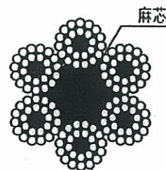
ワイヤーロープ断面図
