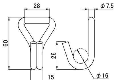
Jフック
