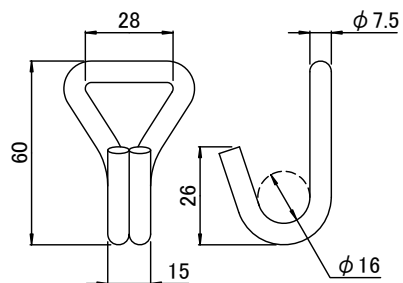
Jフック
