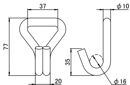
Jフック
