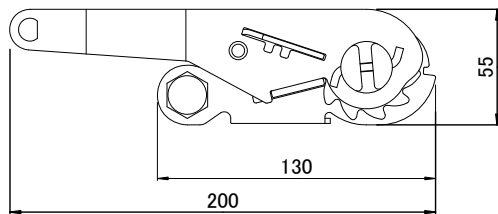
ラチェットバックル
