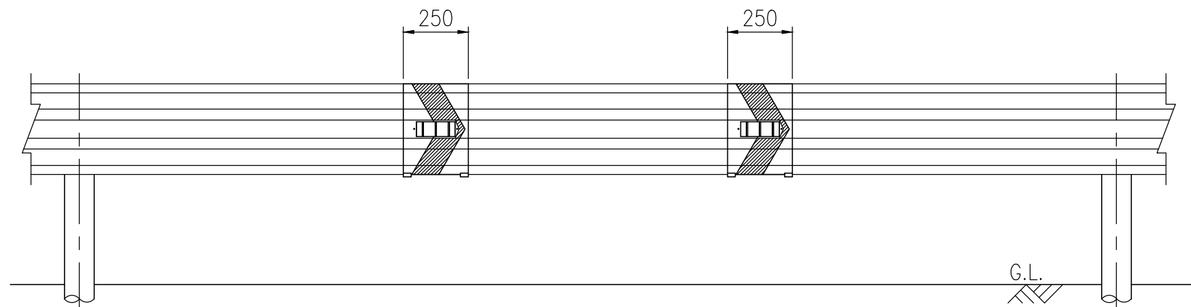
設置図 S=1/20
