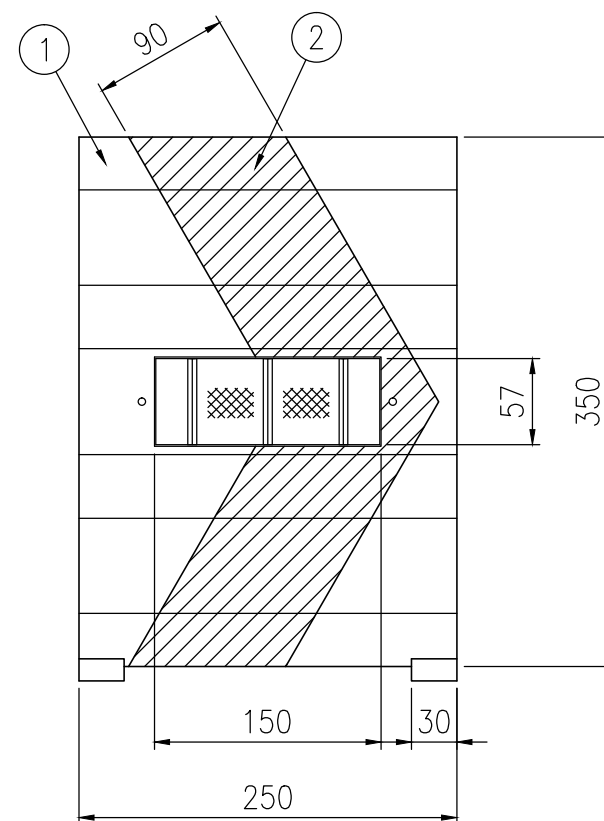
姿図 S=1/5
