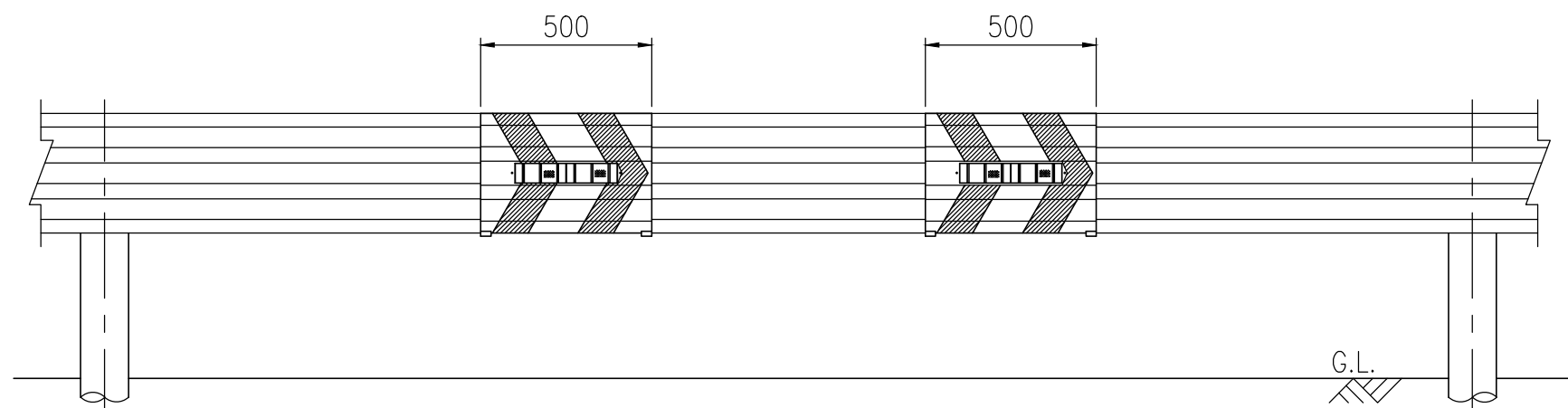
設置図 S=1/20
