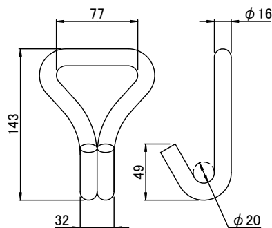
Jフック
