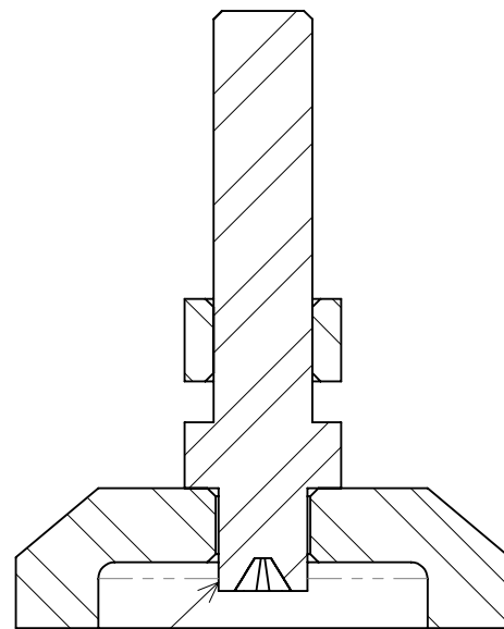
断面図 A-A
