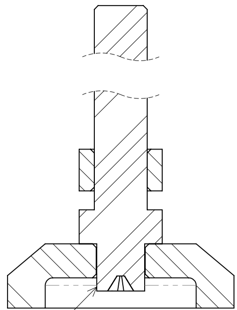
断面図 A-A
