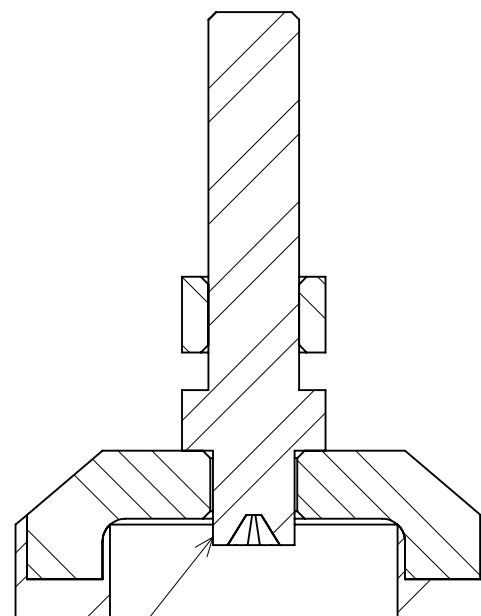
断面図 A-A
