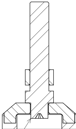
断面図 A-A
